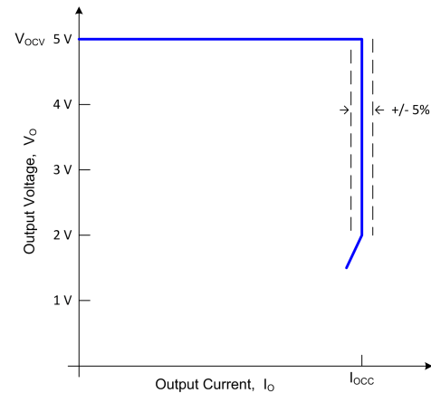
典型伏安图
