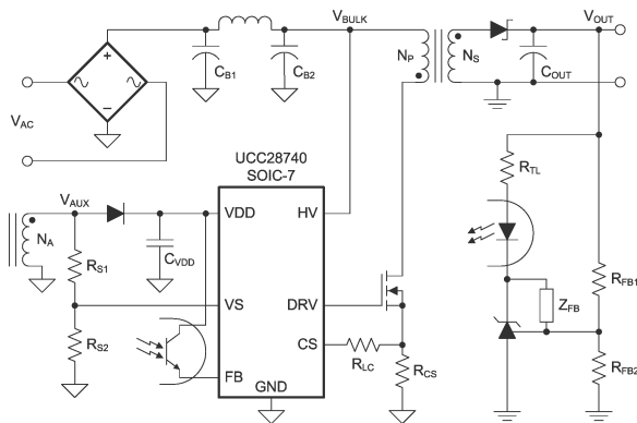
简化应用示意图
