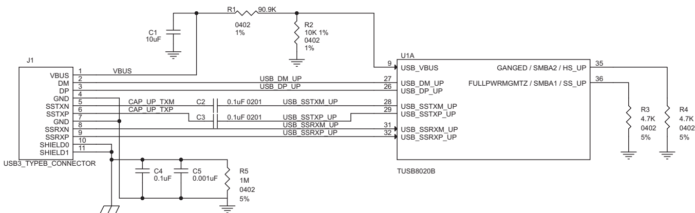
图 27. Upstream Port Implementation
