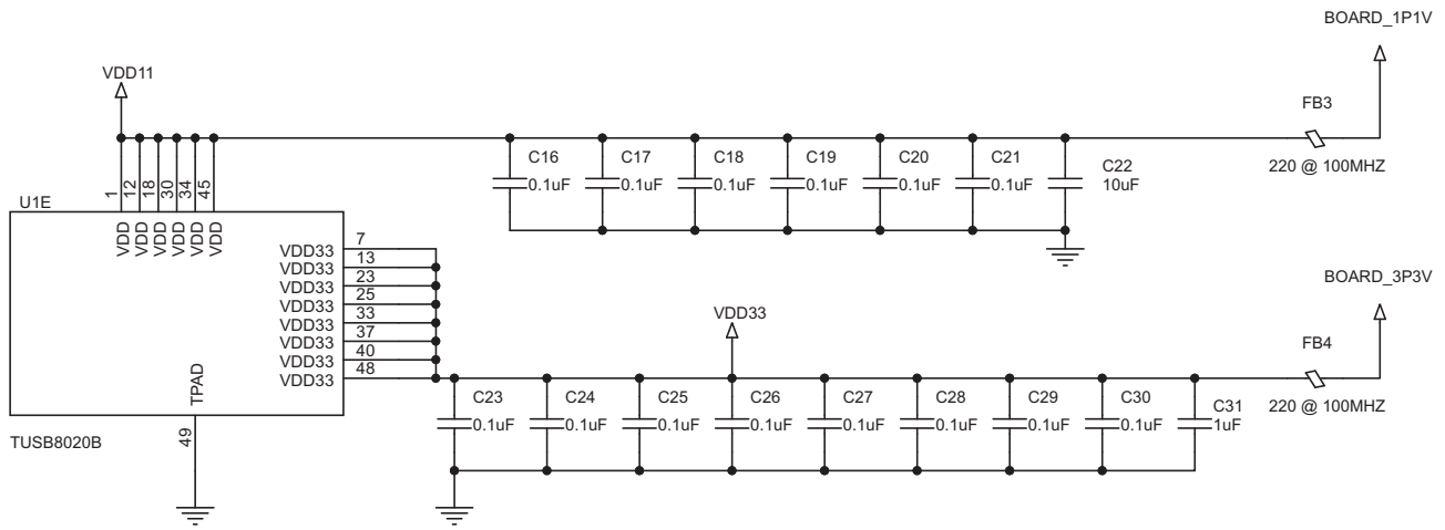
图 32. Power Implementation
