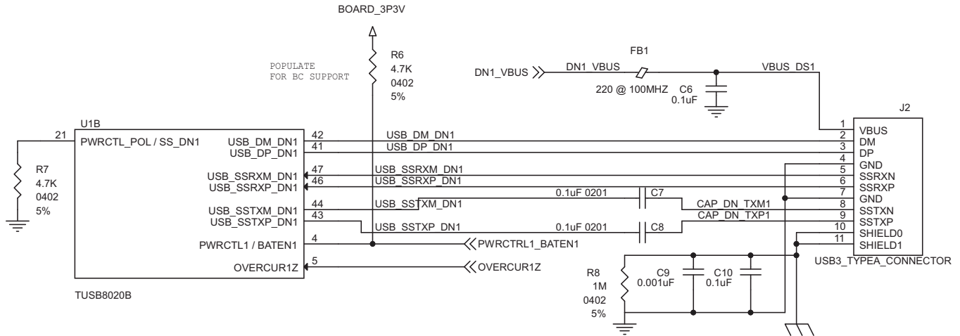
图 28. Downstream Port 1 Implementation
