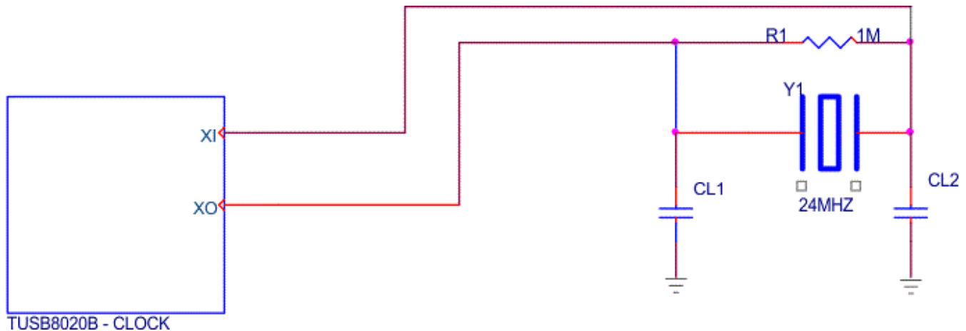
图 2. TUSB8020B Clock
