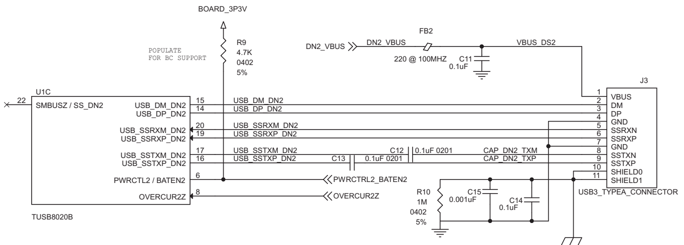
图 29. Downstream Port 2 Implementation
