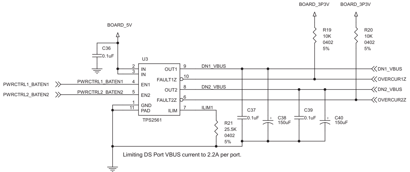
图 30. Power Switch Implementation
