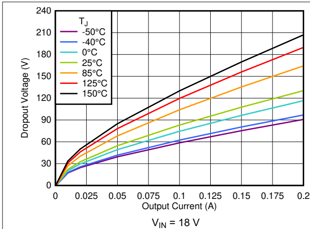
图 6-7. Dropout Voltage vs I_{OUT}
