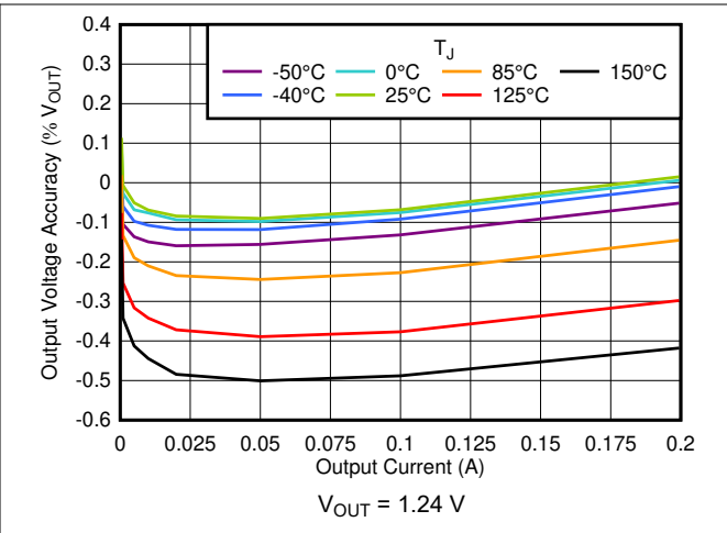
图 6-2. Load Regulation vs I_{OUT}
