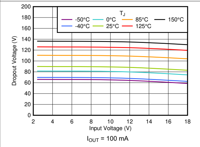
图 6-4. Dropout Voltage vs V_{IN}
