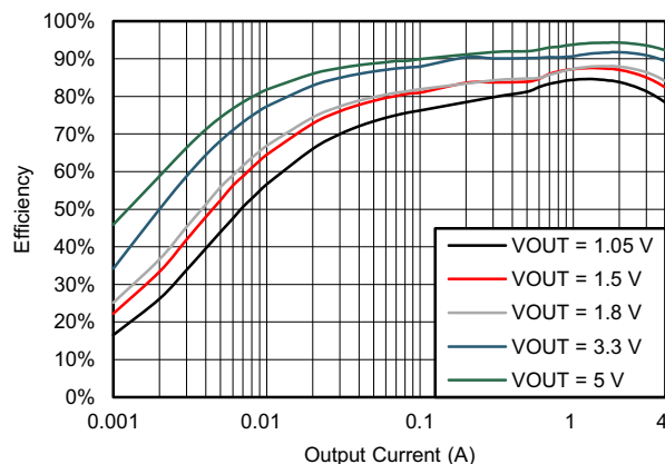
TPS564201 效率
