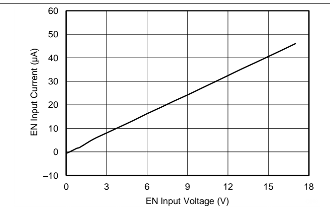
Figure 13. En Current vs En Voltage
