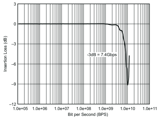
图 6-7. Insertion Loss
