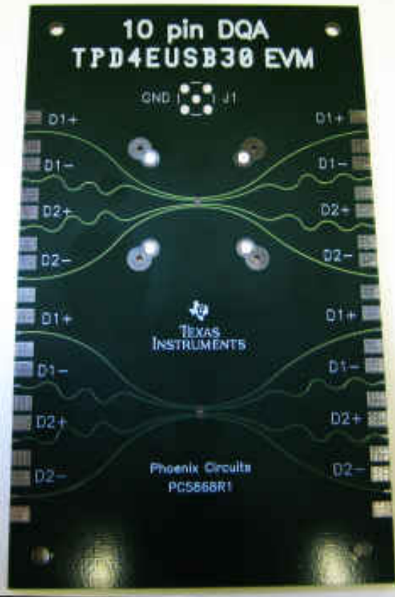
图 10-2. TPDxUSB30/A EVB - TPD4EUSB30 Side
