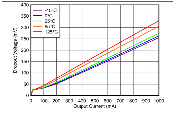
图 15. 5.0-V Dropout Voltage vs I_{OUT}
