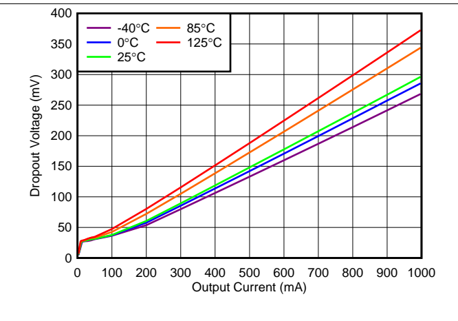
图 14. 3.3-V Dropout Voltage vs I_{OUT}
