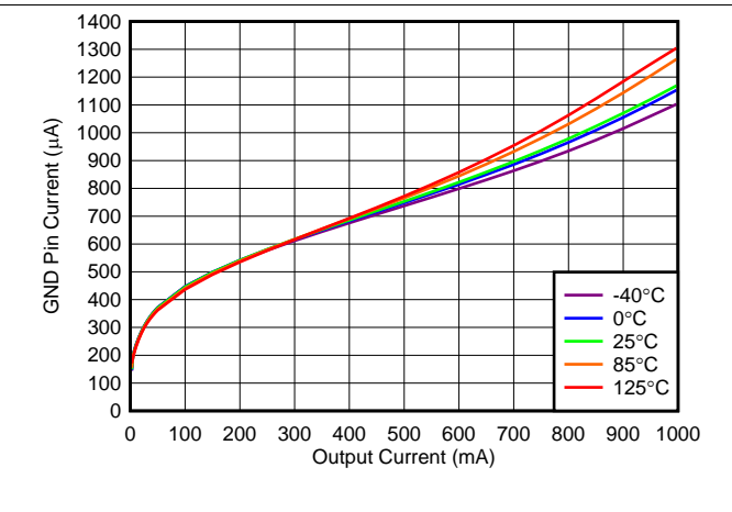
图 18. I_{GND} vs I_{OUT}
