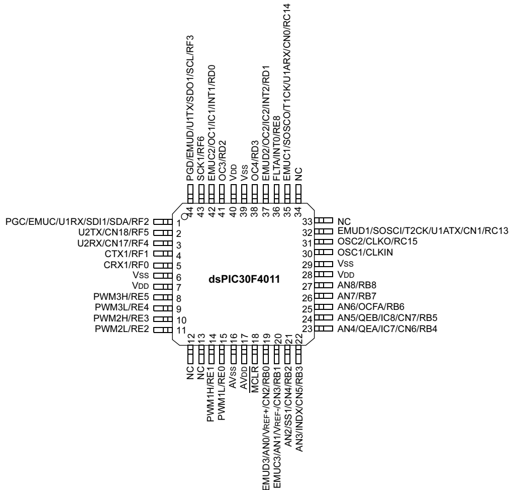
44-Pin TQFP
