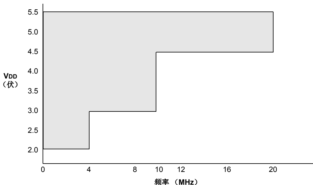
图 12-1: PIC16F630/676 (A/D 关闭时) 的电压 - 频率曲线图, -40^{\circ}\text{C} \leq T_A \leq +125^{\circ}\text{C}
