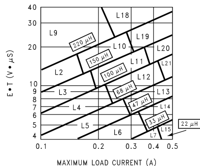
Figure 13. LM2671-ADJ
