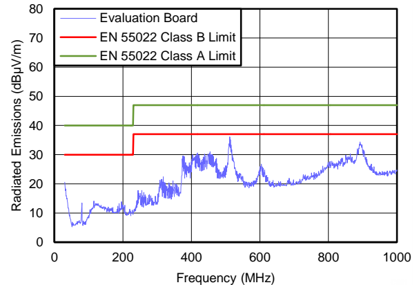
辐射电磁干扰 (EMI) (CISPR22) V_{IN} = 5.0V 、 V_{OUT} = 1.8V 、 I_{OUT} = 1A
