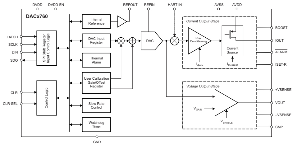
框图
